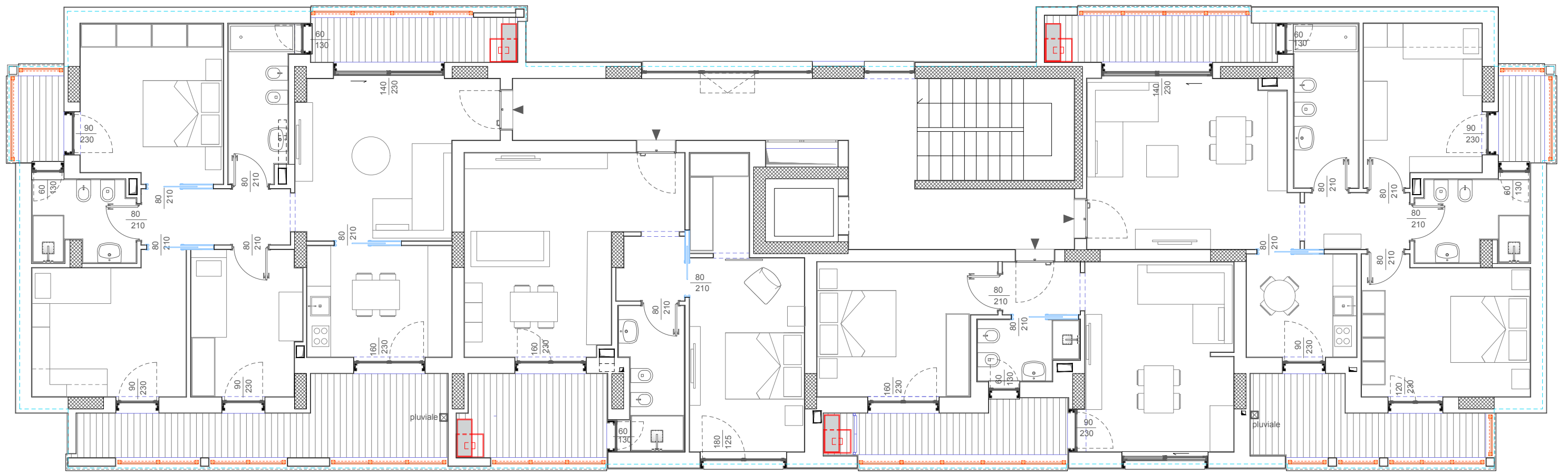
pianta piani secondo - quarto - sesto sc. 1:100
